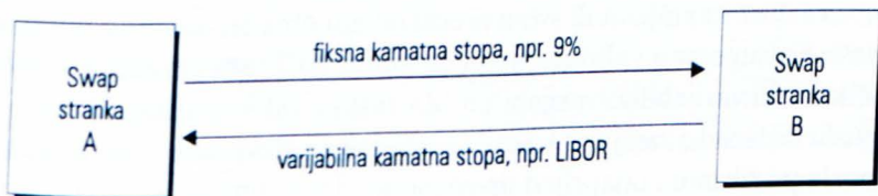
Slika 1. Kuponski swap
