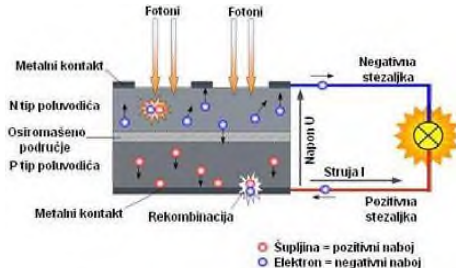
Slika 57.: Fotonaponski efekt
