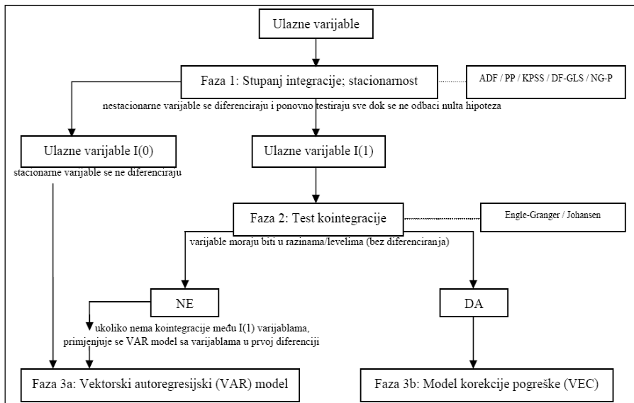
Shema 3. Standardni redosljed postupaka za utvrđivanje kauzalnosti među varijablama
