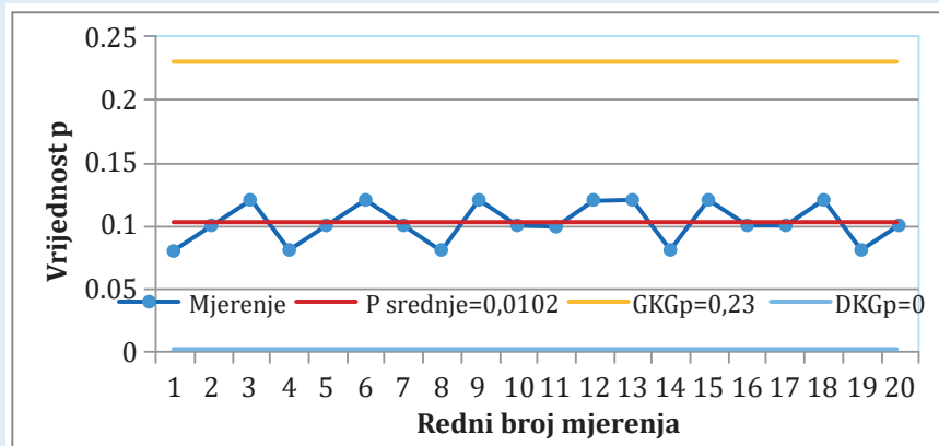
Slika 11.6. p - kontrolna karta
